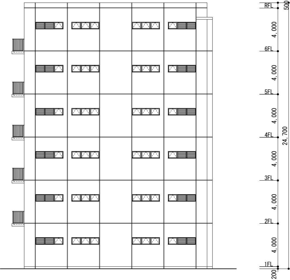
北立面図
