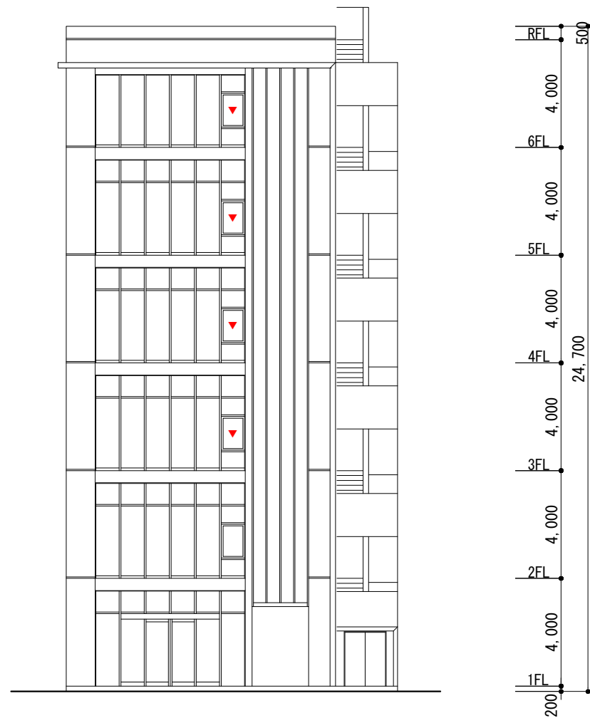
西立面図 S=1:200
