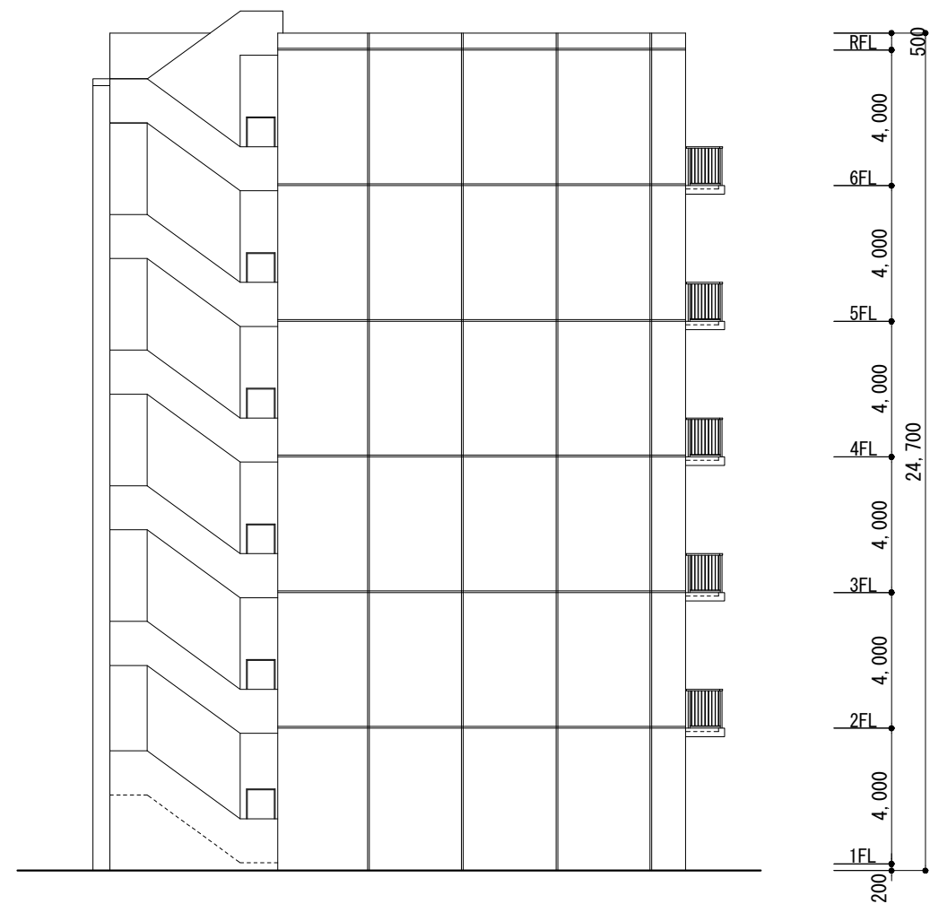
南立面図 S=1:200
