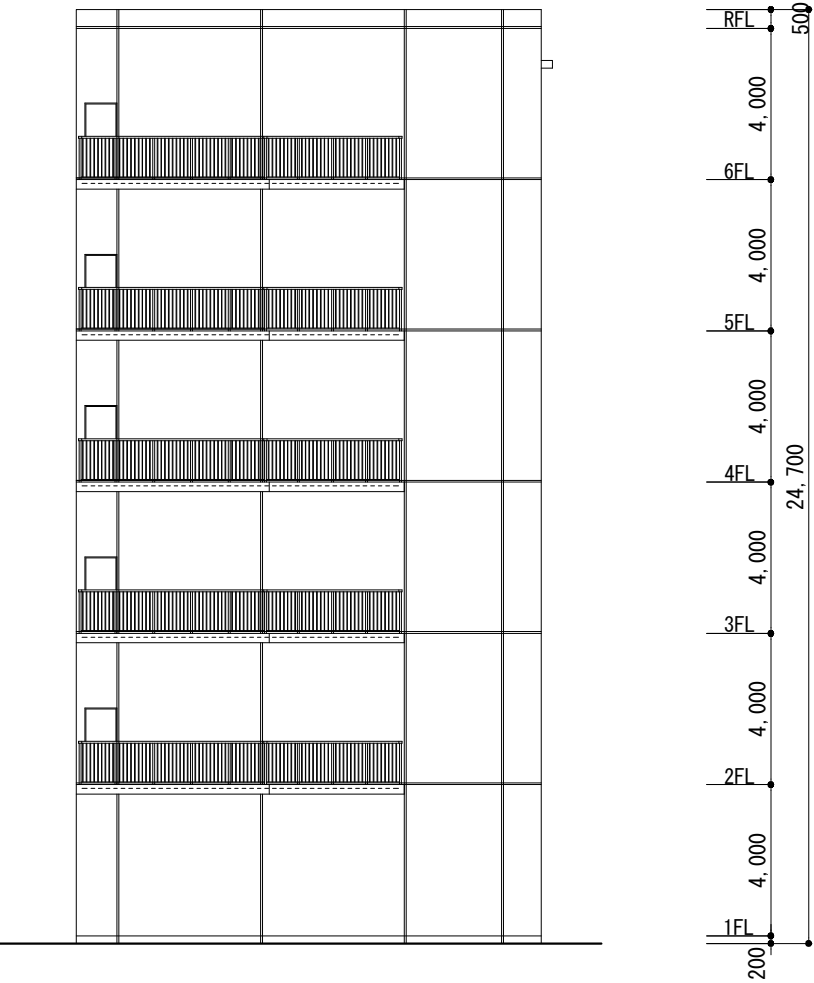
東立面図
